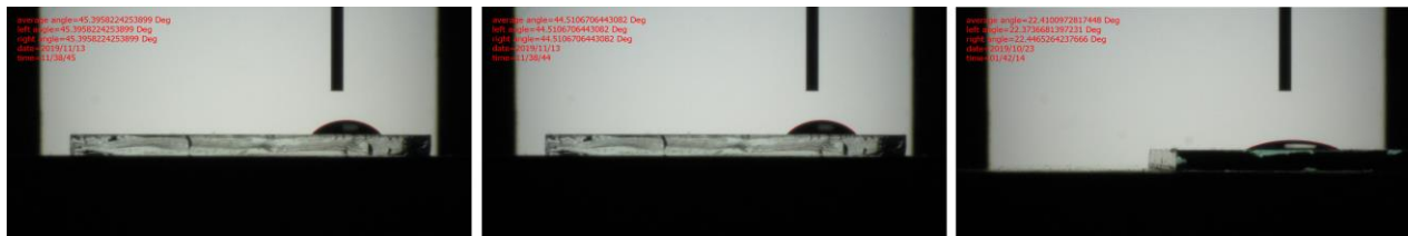
شکل 5- تصاویر زاویه تماس شیشه ی رسانای FTO حاوی لایه های نازک قرار گرفته شده بر روی آن، تهیه شده از کوپلیمر های بلوکی در شرایط مختلف (از چپ به راست دمای تثبیت افزایش می یابد)
