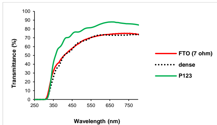
شکل 4- طیف عبوری شیشه ی رسانای FTO و لایه های نازک قرار گرفته شده بر روی آن، تهیه شده از کوپلیمر بلوکی
